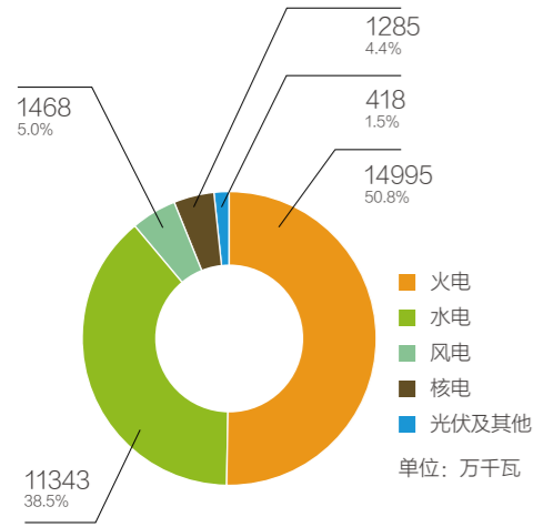
2016年南方五省(区)电源结构
